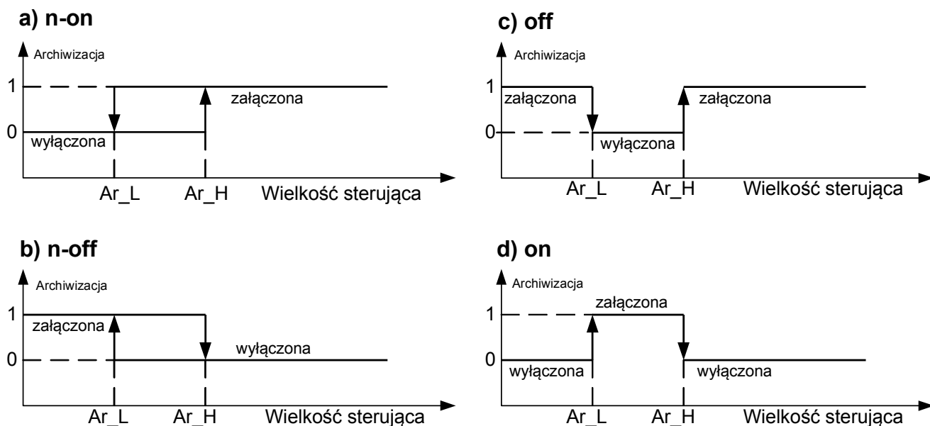
Rys.24. Typy archiwizacji warunkowej
